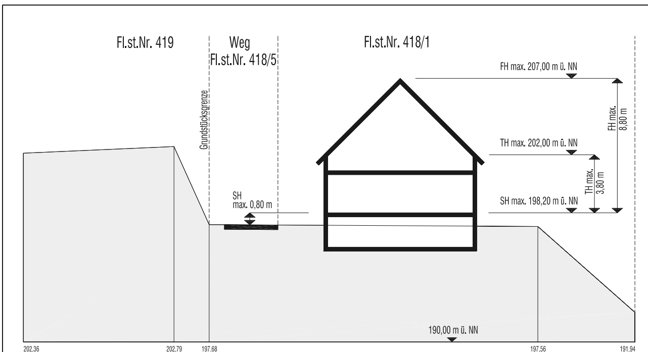
Schnitt I - I
