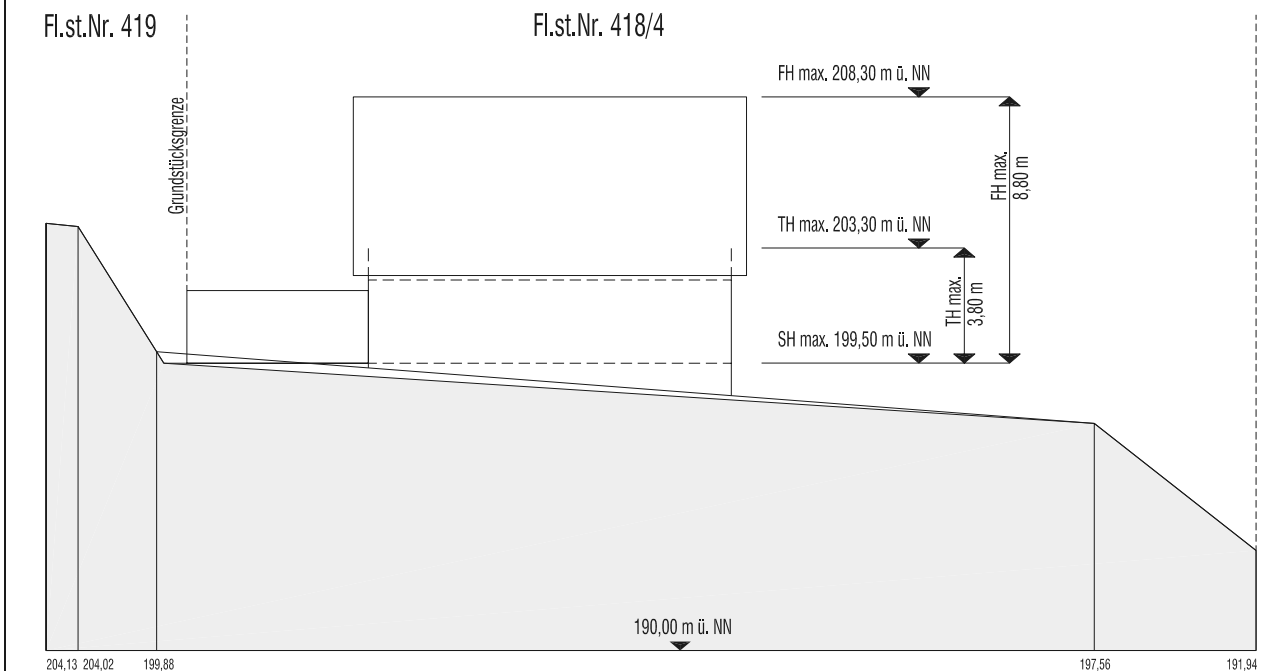
Schnitt II - II
